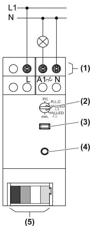
Bilde 2: Koblings skjema
