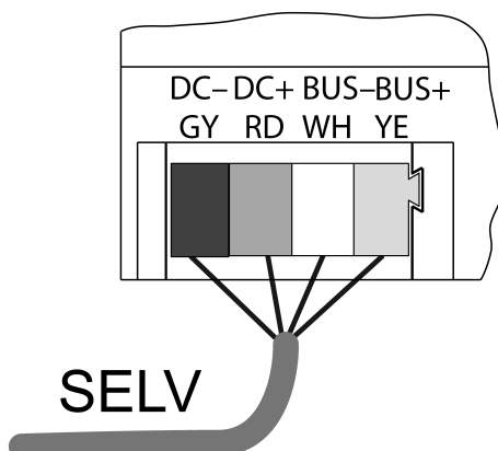
Bilde 1: Koblings skjema bussledning
