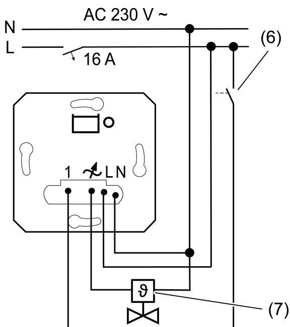
Bild 3: Anslutningsplan i kombination med rumstemperaturregulator-påbyggnad
