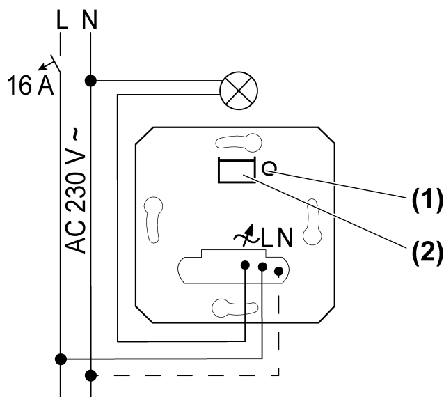
рисунок 1: Монтажная схема
