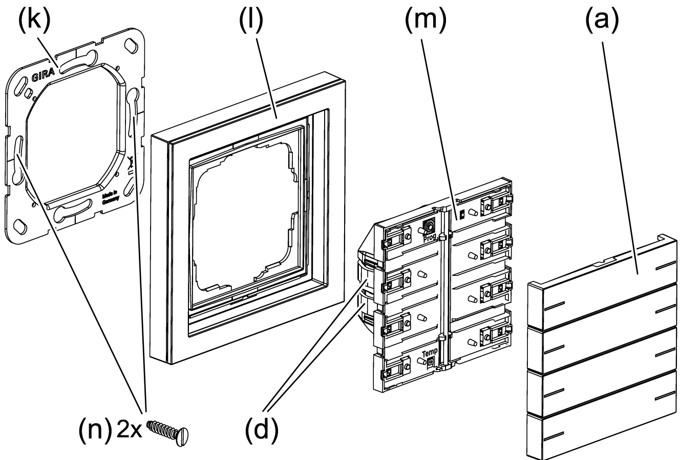
Bild 6: Gerät montieren
