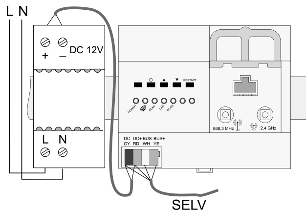
Afbeelding 3: Aansluitschema
