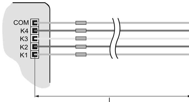
Bild 2: Max. ledningslängd
