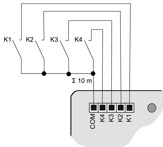
Bild 3: Anslutningsexempel 4-kanals
