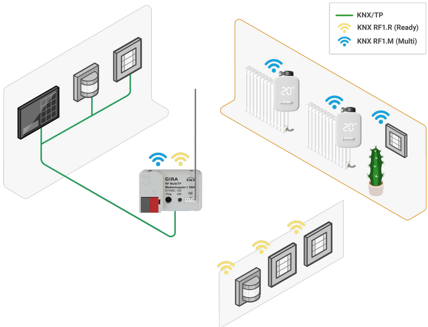
Bild 1: System Gira RF Multi Stellantrieb für KNX
