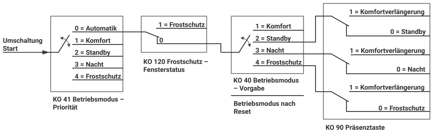
Bild 8: Umschaltung durch KNX Objekt mit Präsenztaste
