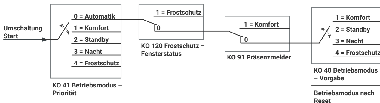
Bild 9: Umschaltung durch KNX Objekt mit Präsenzmelder
