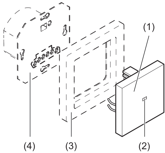
图像 1: 设备结构，单控
