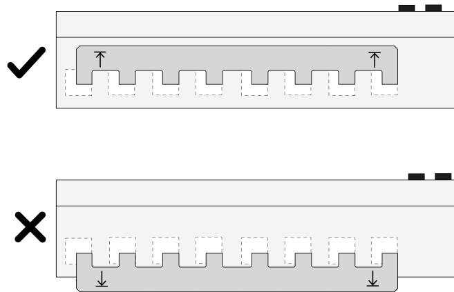
Figura 6: Installazione della sbarra di fase
