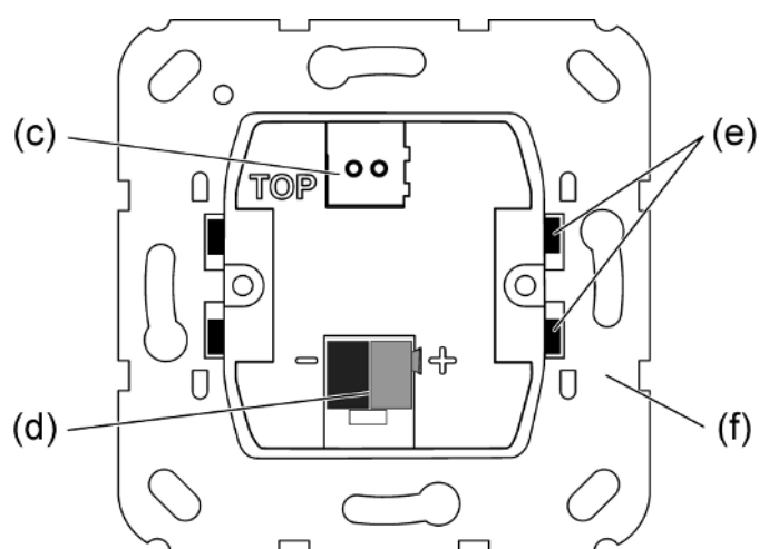
Bilde 3: Apparatets oppbygning - bakside
