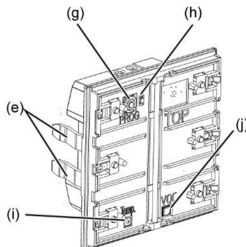
Bilde 4: Tastsensor
