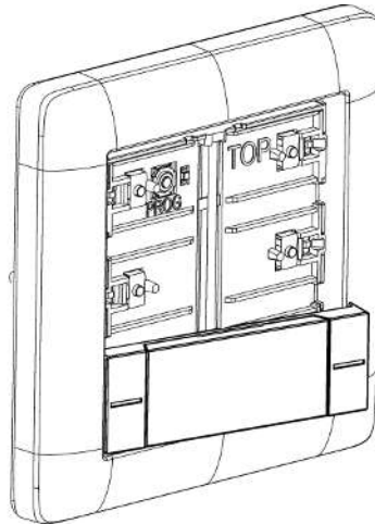
Bilde 6: Installere vippestasten på siden
