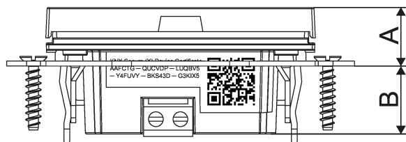
Imagen 11: Dimensiones de montaje
