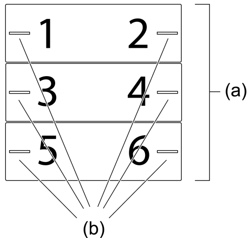
Imagen 1: Estructura del aparato triple (posición de montaje "estándar", interruptores basculantes de mando horizontales)
