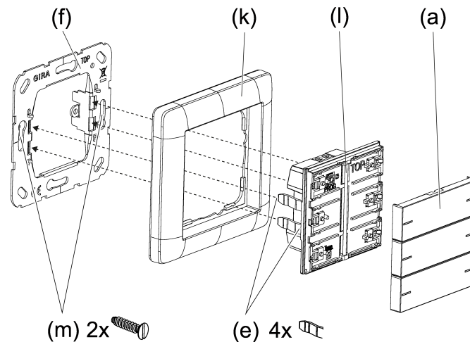
Imagen 5: Montar el aparato
