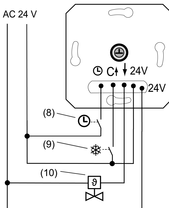
Bild 2: Anslutningsexempel för insatsen
