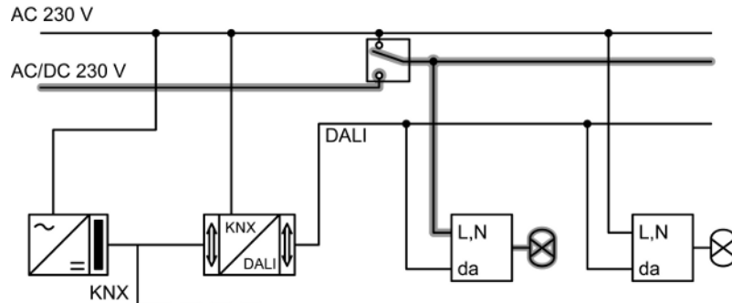
Bilde 3: Nødlamper forsynt av den sentrale sikkerhetsforsyningen
