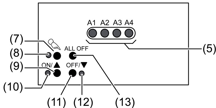
Bilde 3: Betjeningsselementer
