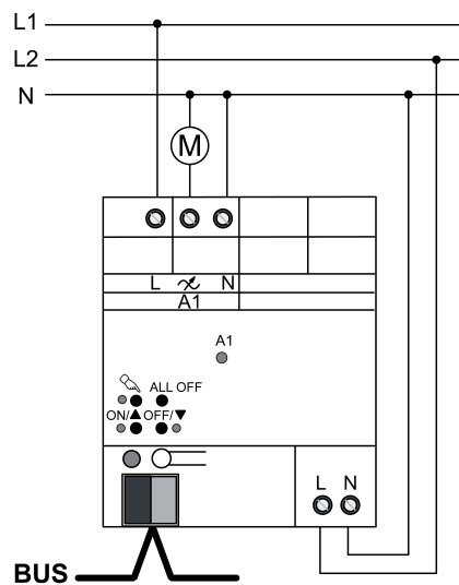
Bild 6: Dimmaktor 1fach – Anschluss für Drehzahlstellerbetrieb
