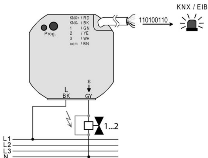
Bild 26: Kurzschluss- und Überlasterkennung bei Störung des Ventilausgangs oder Ventilantriebs
