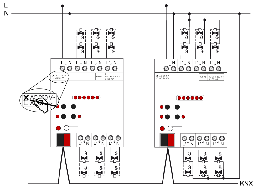
Bilde 3: Tilkobling for ventilaktuator AC 230 V (tilkoblingseksempler) venstre: Nøytrallederne for ventilaktuatorerne føres separat til aktuatoren / høyre: Felles nøytralleder for ventilaktuatorer
