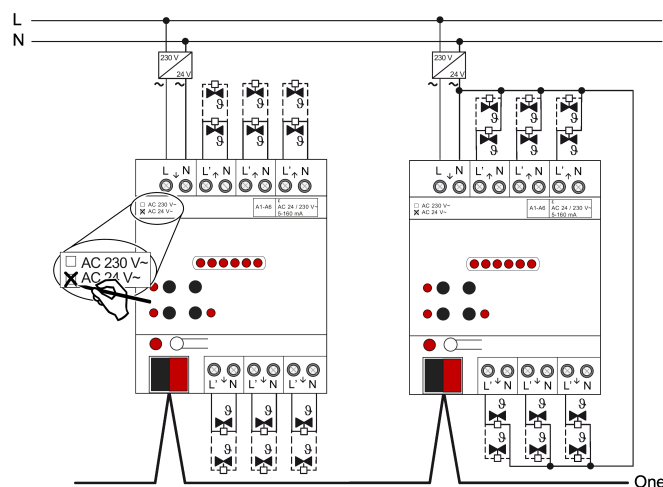
Afbeelding 4: Aansluiting voor ventilaandrijvingen AC 24 V links: gescheiden aansluiting van de ventilaandrijvingen afzonderlijk aan de actor rechts: gemeenschappelijke draad voor ventilaandrijvingen
