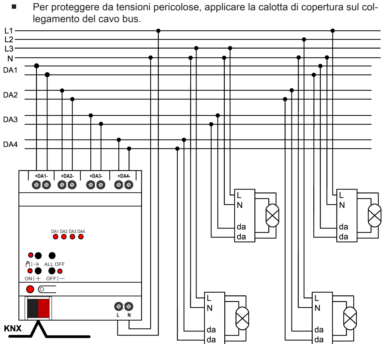
Figura 2: Esempio di collegamento
