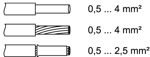
Bild 4: Klemmbare Leitungsquerschnitte
