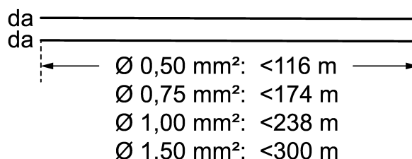
рисунок 4: Длина провода DALI
