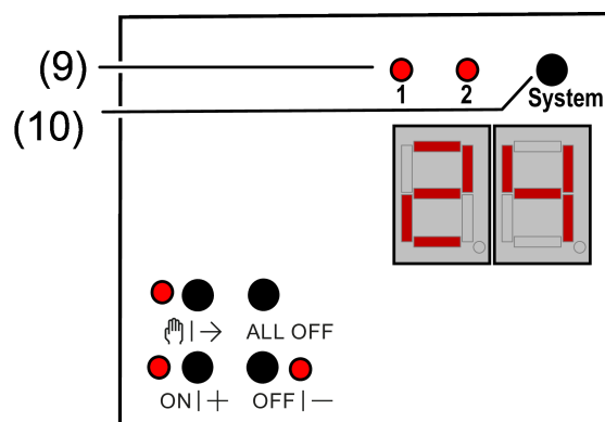
рисунок 2: Панель управления 2-канальным шлюзом DALI
