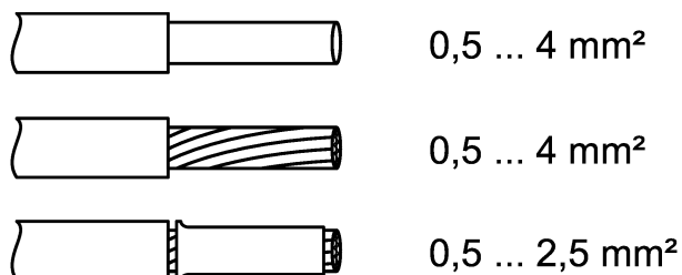
рисунок 5: Поперечные сечения проводов, на которые могут устанавливаться зажимы
