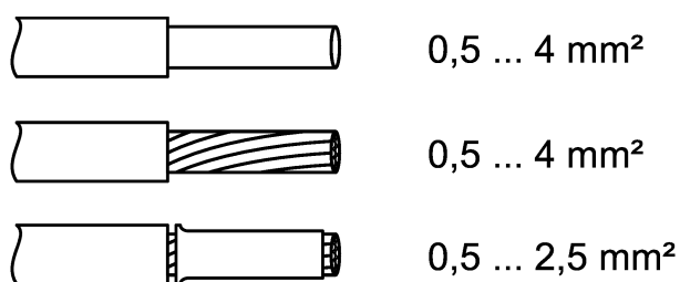
Bilde 5: Klembare kabelverrsnitt
