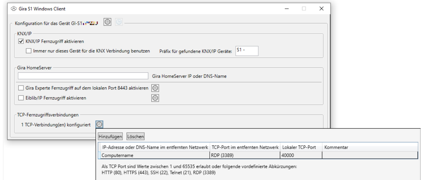
Bild 35: TCP Fernzugriffskonfiguration
