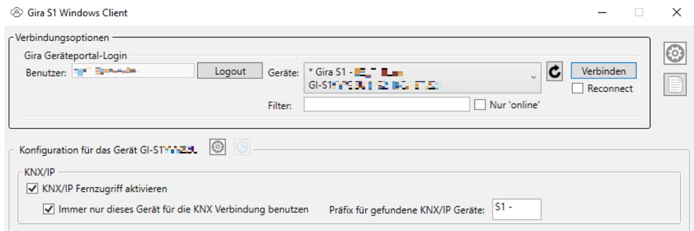
Bild 31: KNX/IP Fernzugriffskonfiguration
