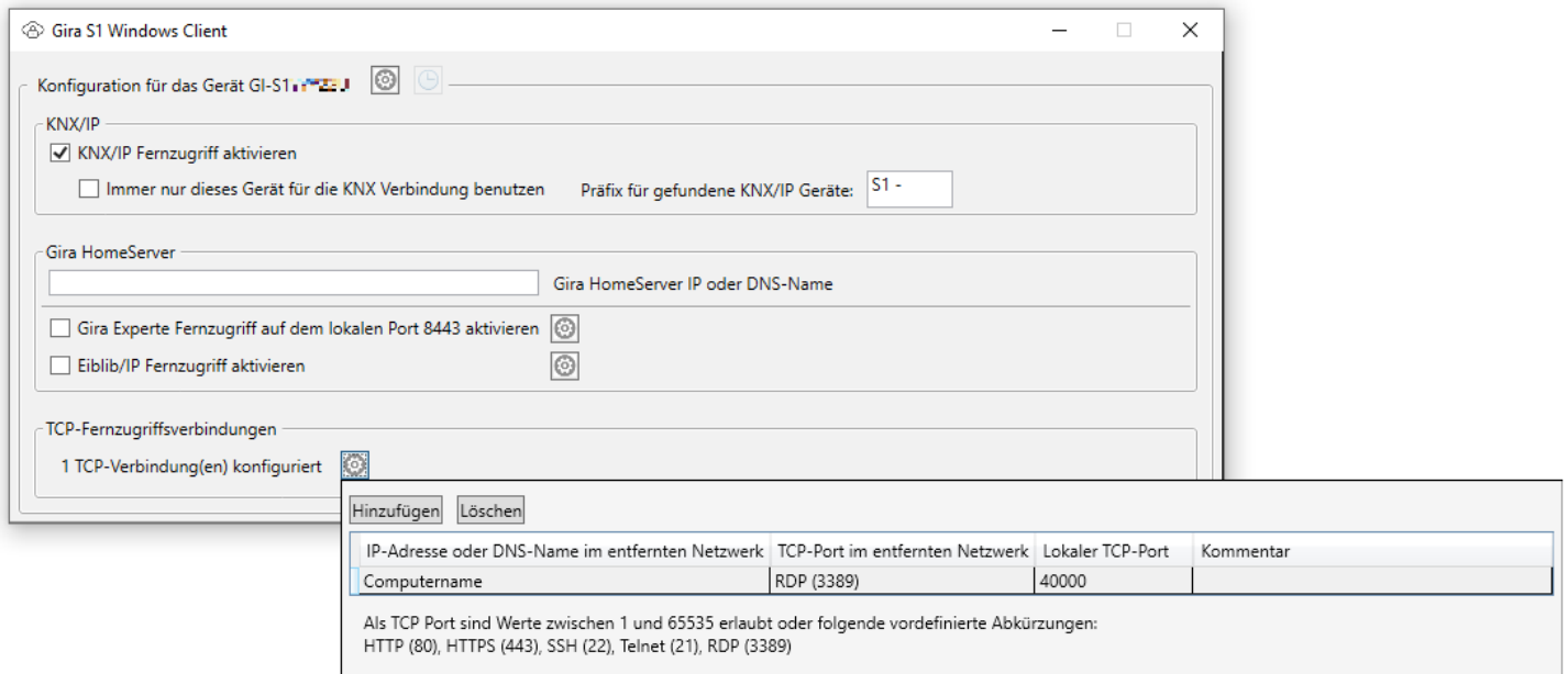
Bild 35: TCP Fernzugriffskonfiguration
