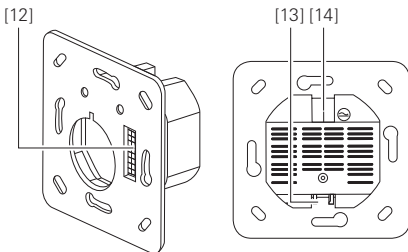
Afb. 4 Inbouwaansluitmodule 24 V
