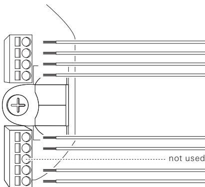
Afb. 10 Kleurcode EIA/TIA568A/B
