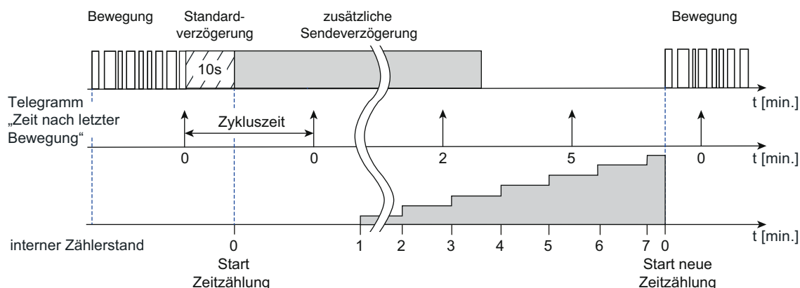
Bild 50: Messung der Zeitspanne nach letzter Bewegung
