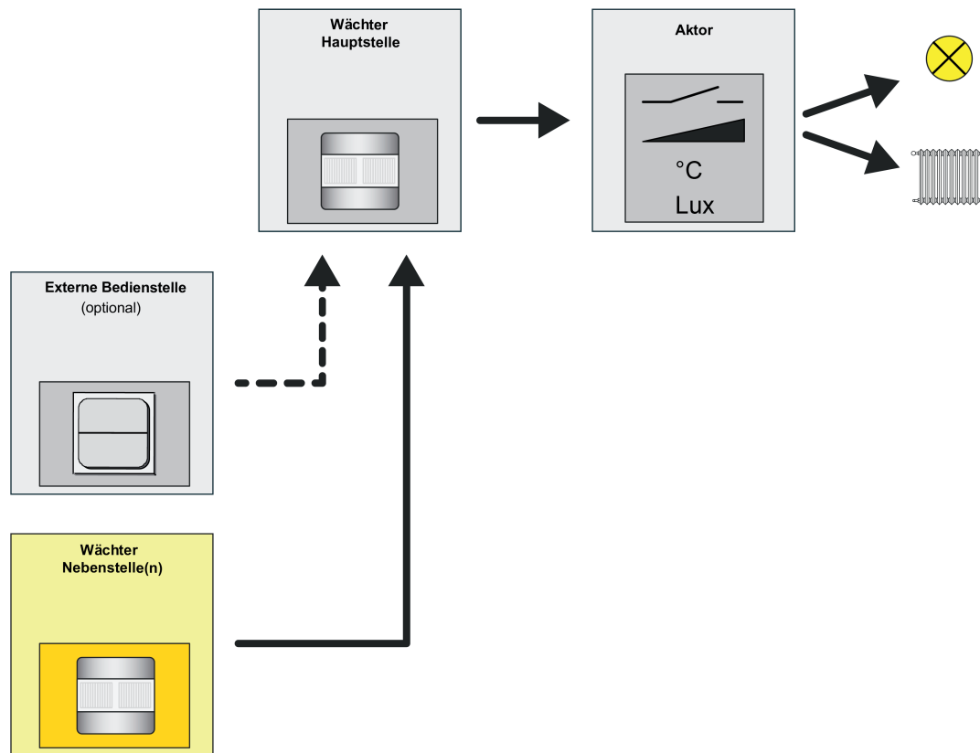
Bild 31: Applikationstyp "Nebenstelle"
