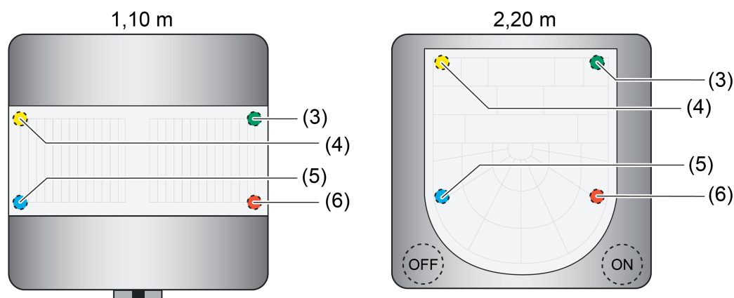
Bild 34: Anordnung der LED zur Anzeige der Betriebszustände
