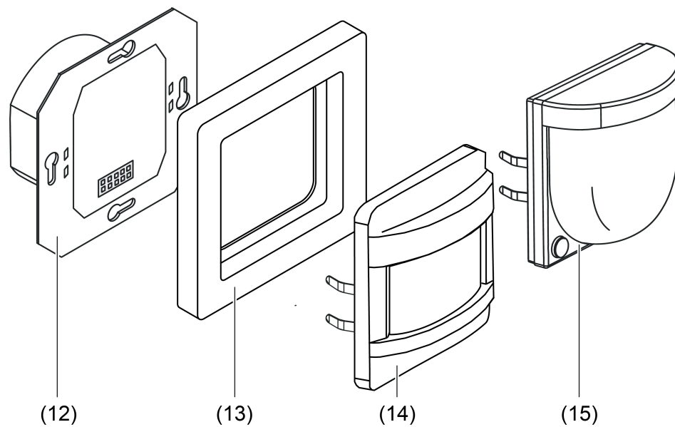
Bild 17: Montage
