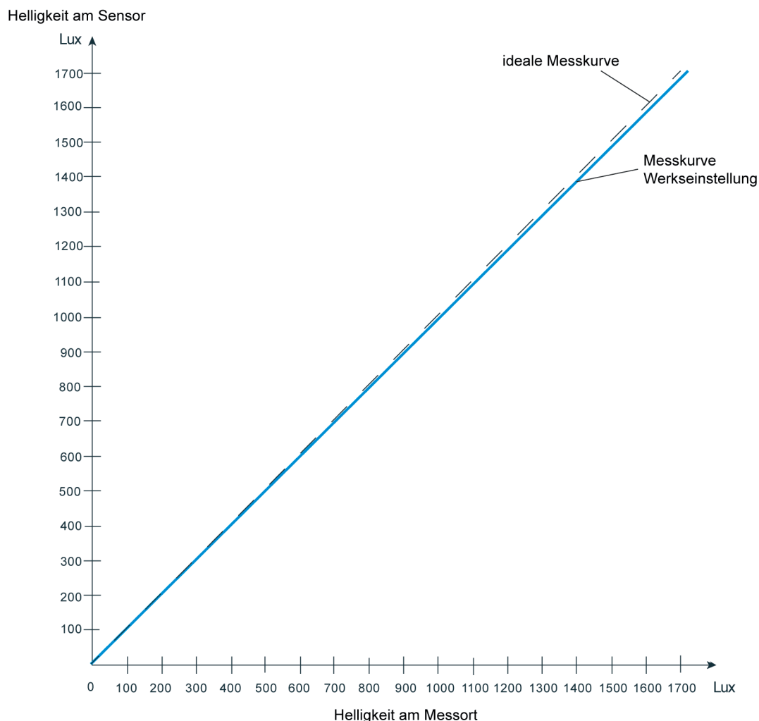
Bild 22: Messkennlinie nach Werkseinstellung (Sensormesswert = Umgebungshelligkeit = ideale Messkennlinie)
