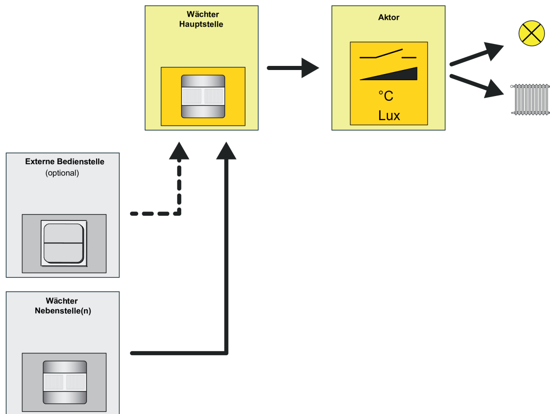
Bild 30: Applikationstyp "Hauptstelle"
