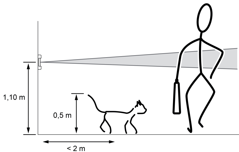
Bild 4: Erfassungsfeld und Einbauhöhe
