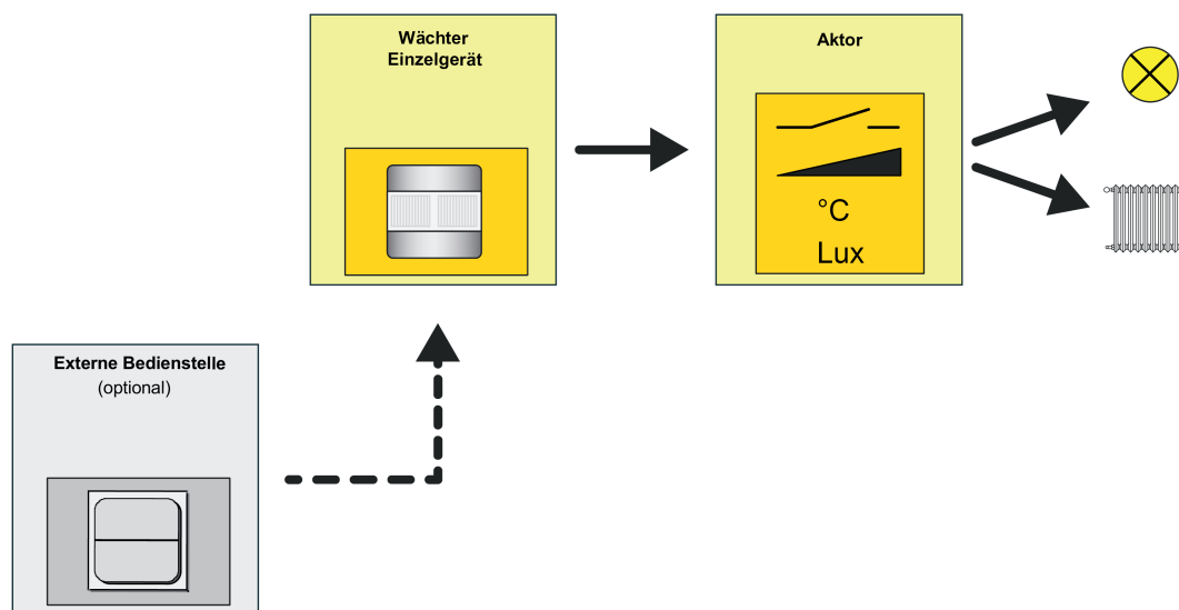
Bild 29: Applikationstyp "Einzelgerät"
