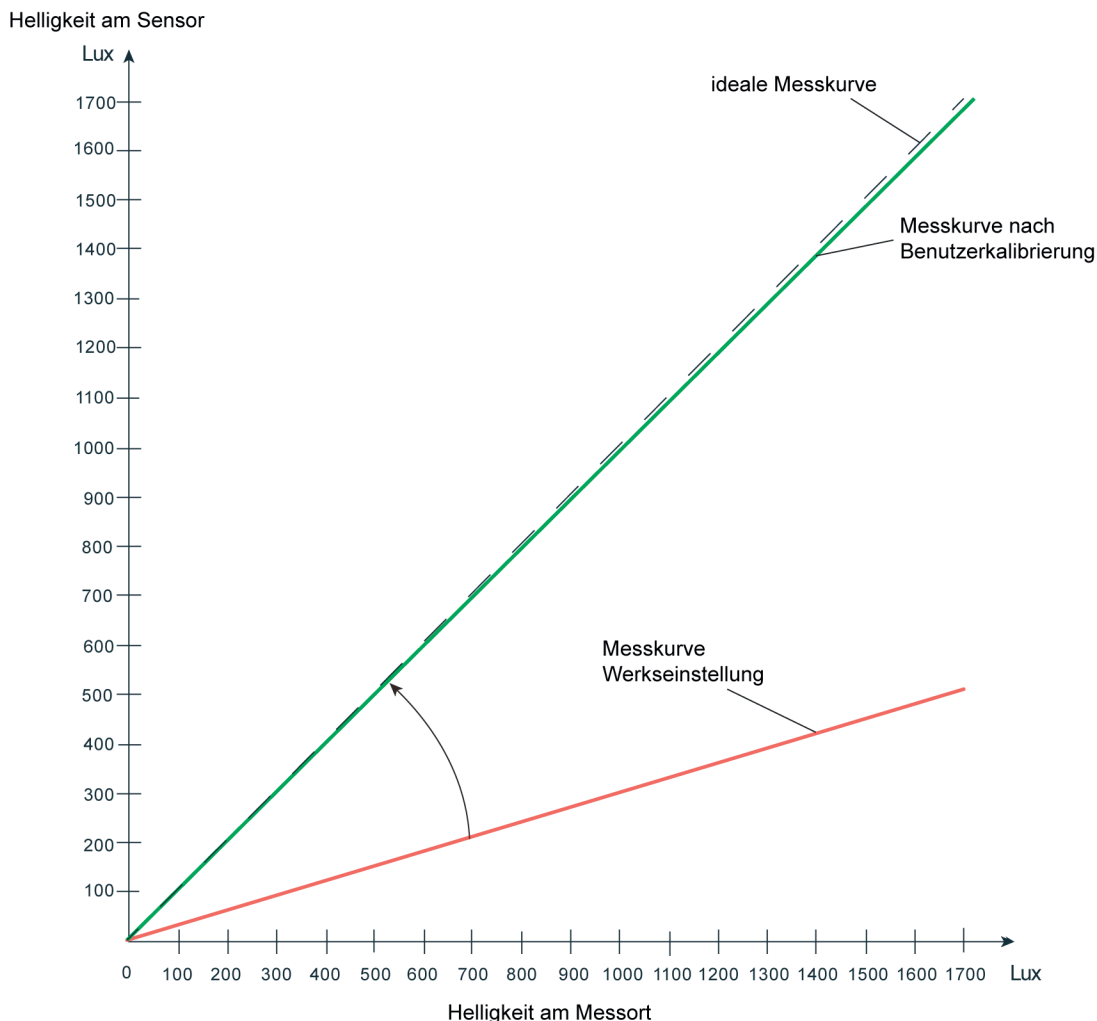
Bild 23: Messkennlinie nach Benutzerkalibrierung (Korrektur des Sensormesswerts auf die Umgebungshelligkeit = ideale Messkennlinie)
