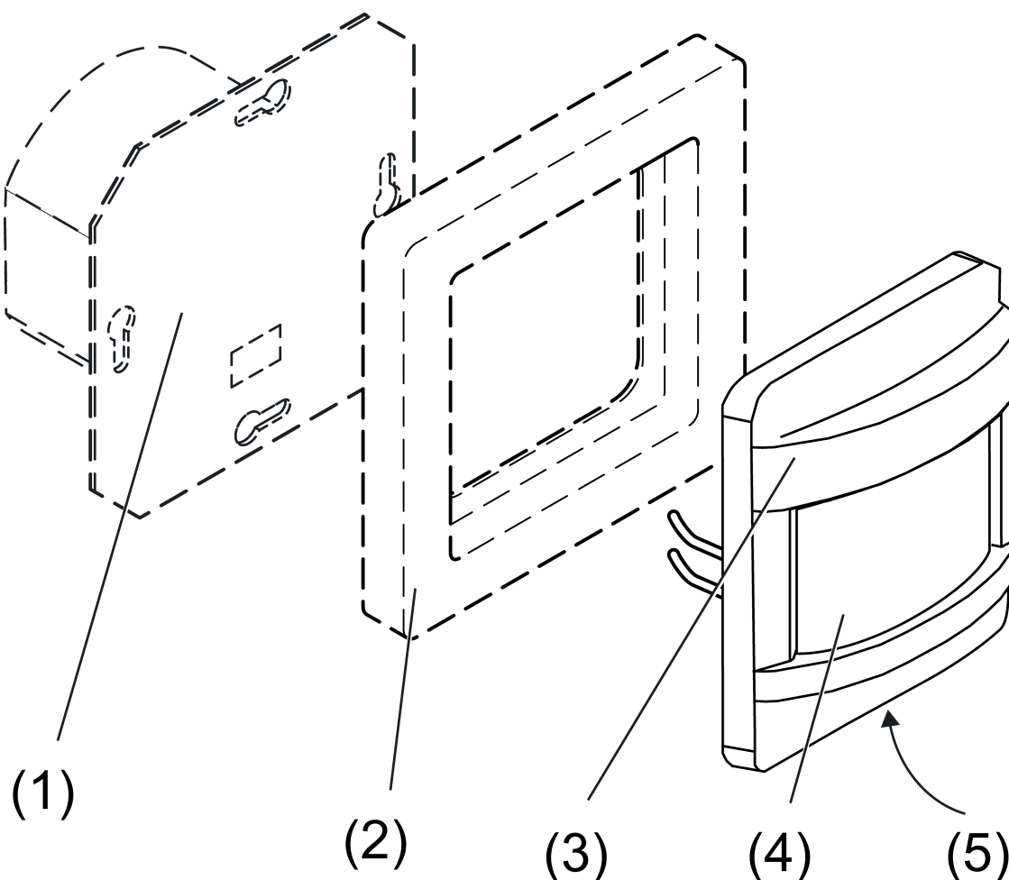
Bild 1: Enhetens konstruktion
