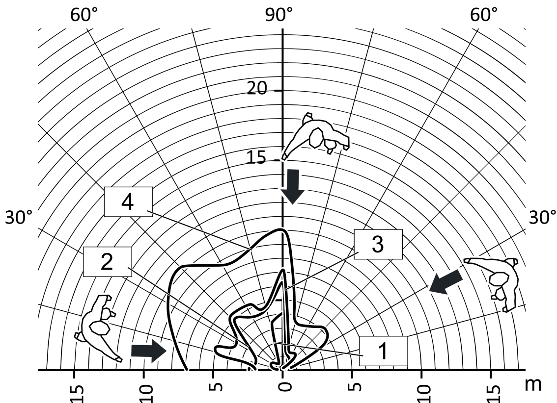
Bild 14: Räckvidd vid radiell rörelseriktning
