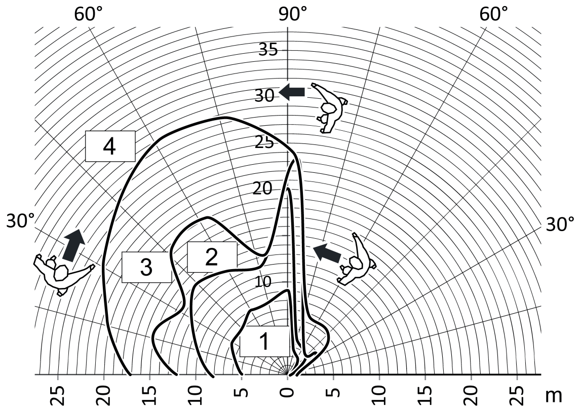
Bild 13: Räckvidd vid tangentiell rörelseriktning
