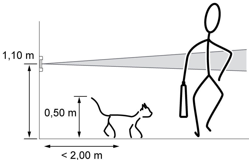
Bild 11: Övervakningsområde och monteringshöjd
