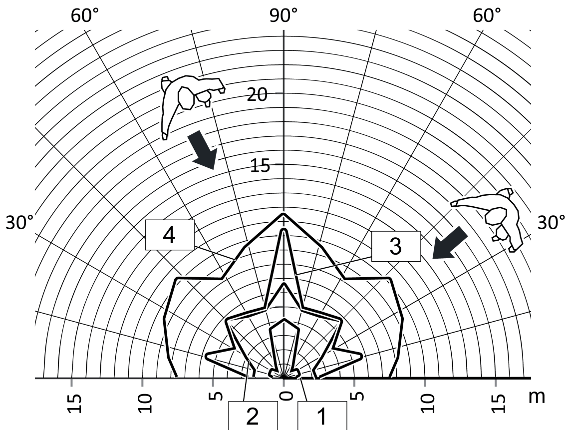
Bild 10: Räckvidd vid radiell rörelseriktning
