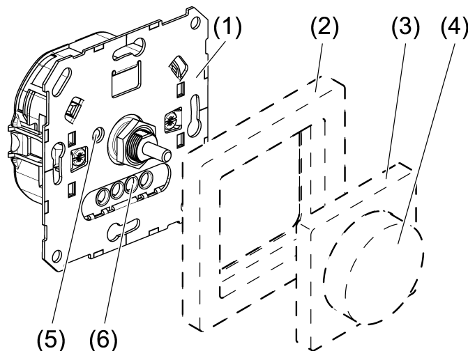
Afbeelding 1: Constructie apparaat
