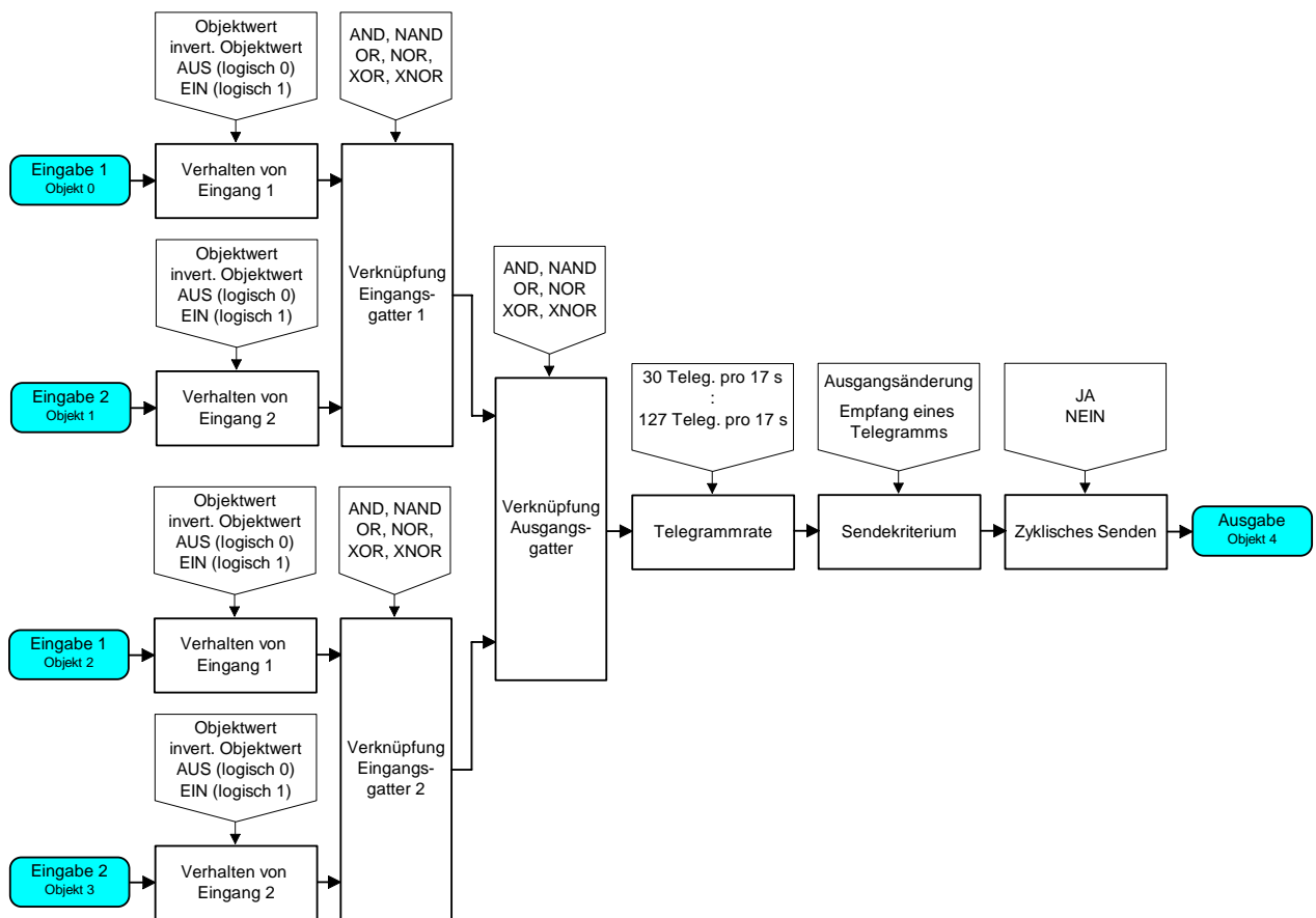
Funktionsschaltbild
