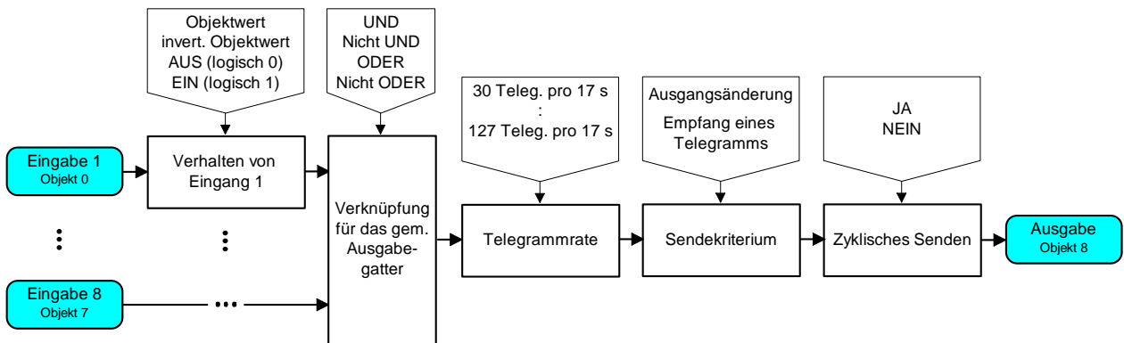
Funktionsschaltbild
