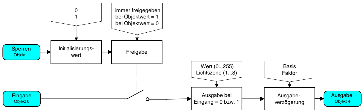
Funktionsschaltbild: Freigabefunktion parametriert
