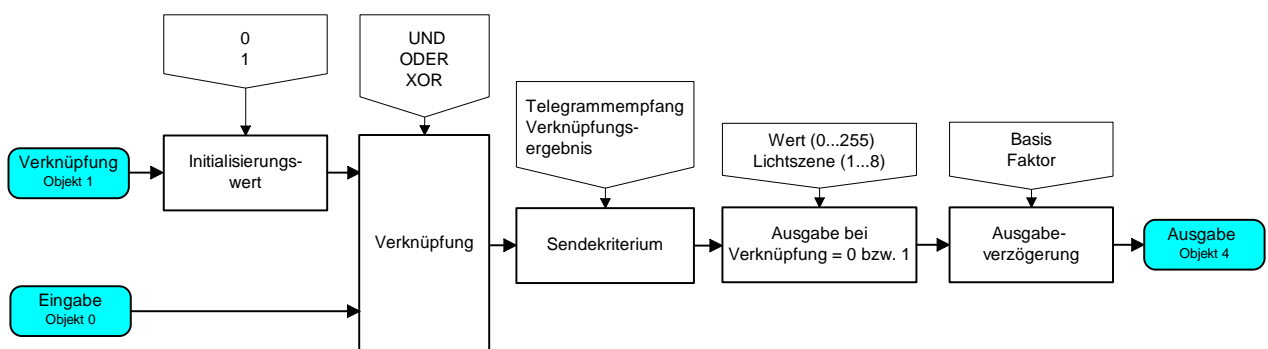
Funktionsschaltbild: Verknüpfungsfunktion parametriert
