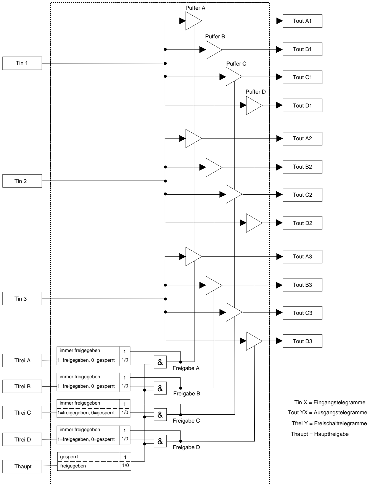
Funktionsschaltbild
