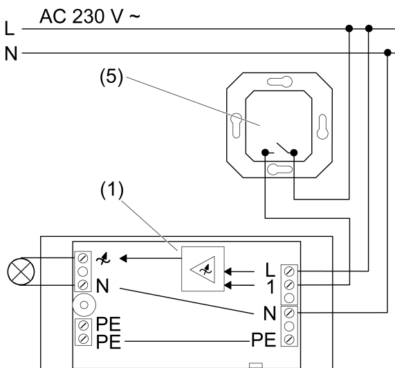
Bilde 5: Koblingsskjema snordimmer med installasjonstast
