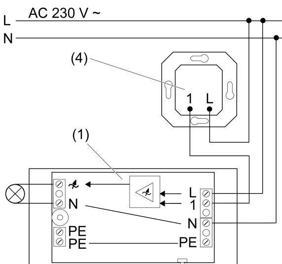
Bilde 4: Koblingsskjema for snordimmer med biapparat totrådsledning
