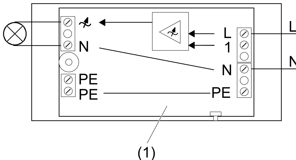
Bilde 3: Koblingsskjema snordimmer
